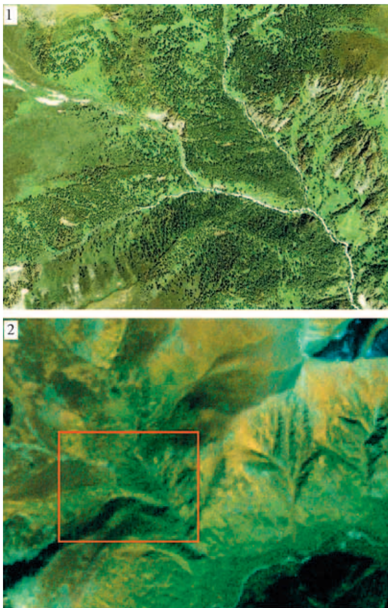
Рис.8. Зависимость дешифровочного признака структура изображения от пространственного разрешения снимка: 1 – GeoEye-1, размер пиксела 2 м, 2 – TM/Landsat 5, размер пиксела 30 м
